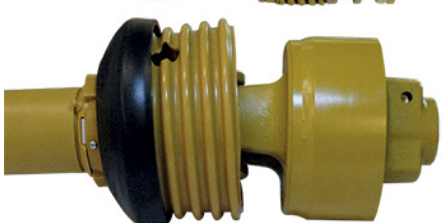
Gelenkwelle mit Nockenschaltkupplung
