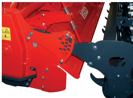
Réglage latéral du rouleau arrière
