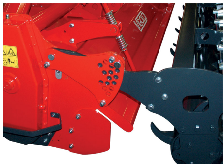
Regolazione laterale dei rulli con perni
