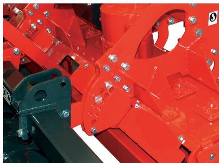
Regolazione laterale dei rulli con perni
